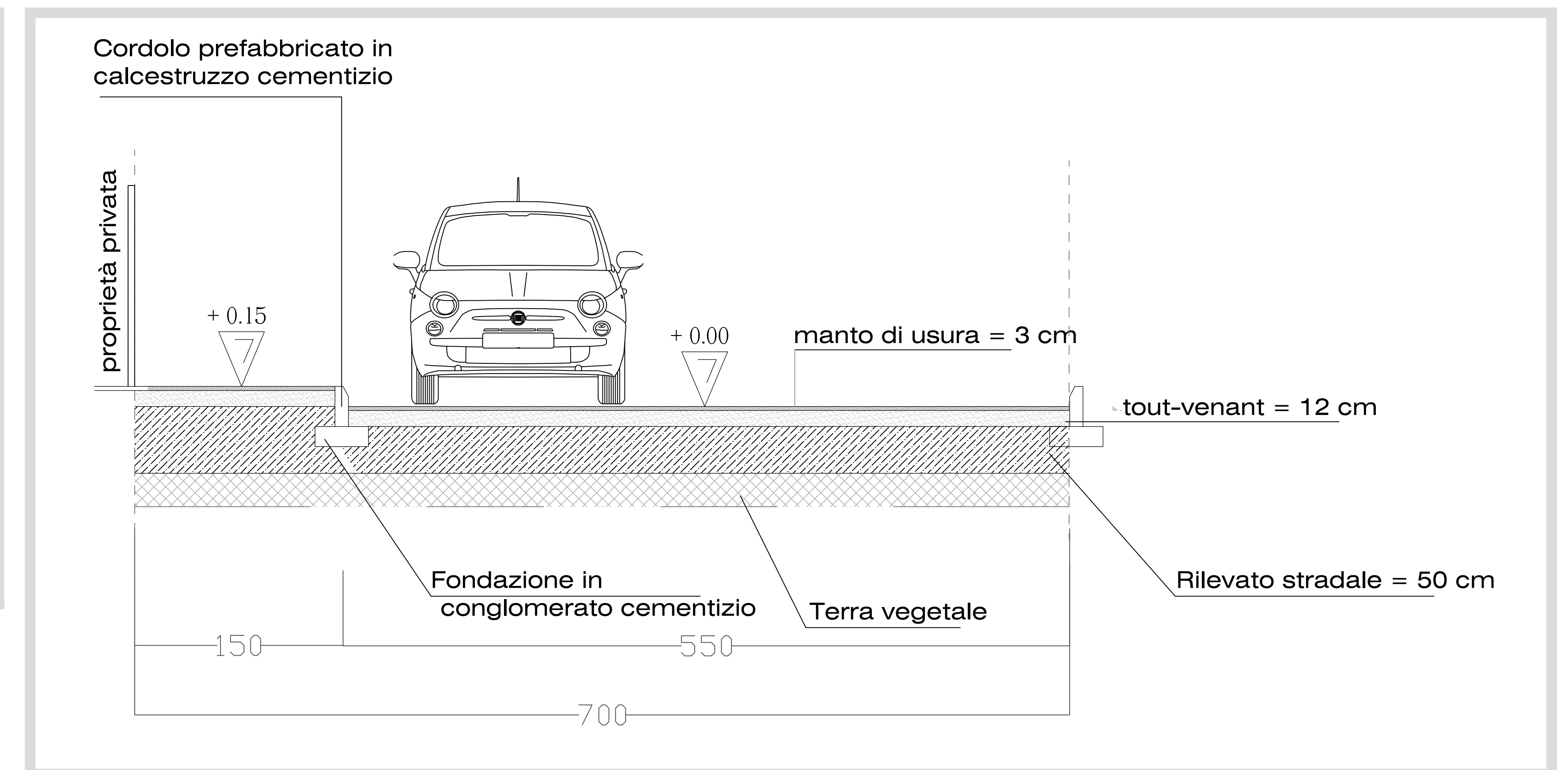
SEZIONE STRADA
