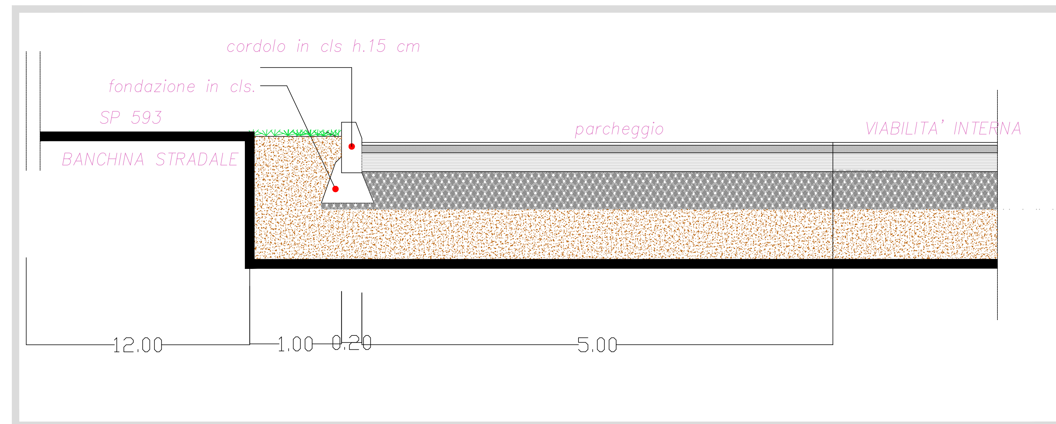
SEZIONE AREA PARCHEGGIO A-A
